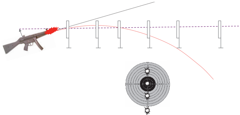
Şekil 3. Nişan hattı ve mermi yolu ilişkisi
