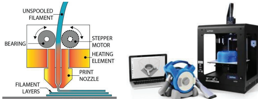
Şekil 1. 3B FDM plastik yazıcı çalışması.
