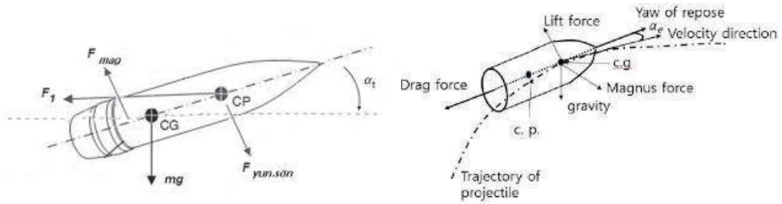
Şekil 1. Dış balistikte mermiye etki eden kuvvetler
