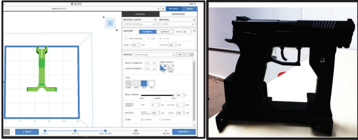
Şekil 3. Silah sabitleme sistem prototipinin montajlanmış görüntüsü.
