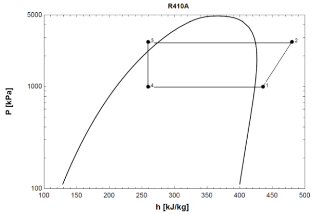
Şekil 2.6 Soğutma çevrimine ait P-h diyagramı
