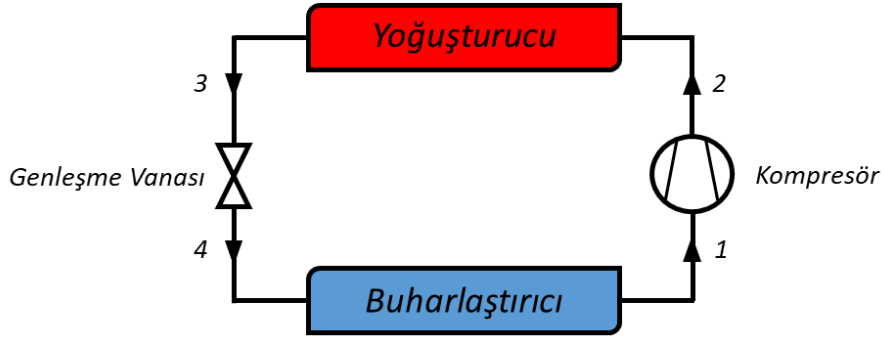
Şekil 2.4 Soğutma Çevrimi
