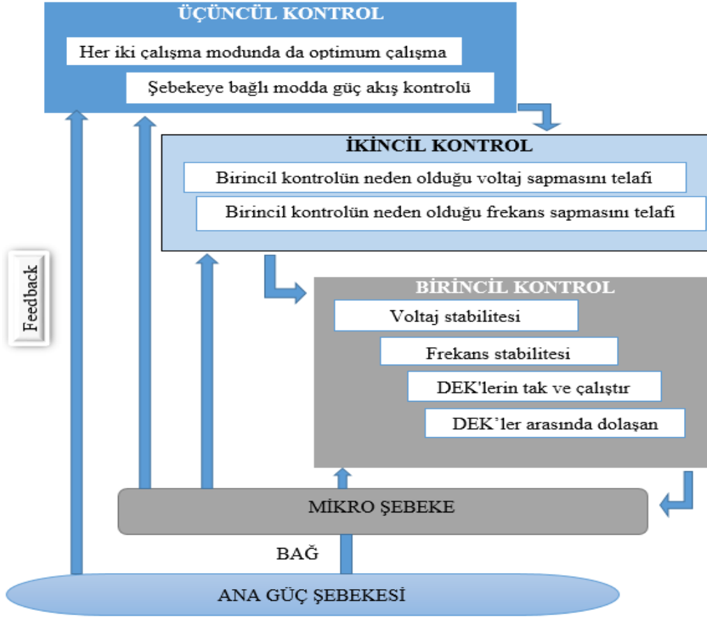
Şekil 2.4 Hiyerarşik kontrol katmanları
