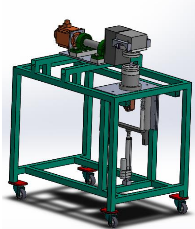
Şekil 2. Simülatör cihaz tasarımının genel görünümü
