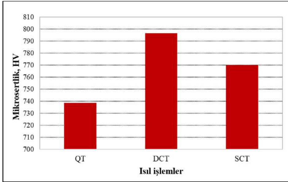
Şekil 5. Farklı ısıtım işlem uygulanmış çelik numunelerin mikrosertlik değışim grafiğı.
