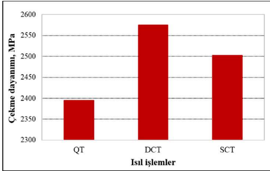
Şekil 6. Farklı ısıt işlem uygulanmış çelik numunelerin çekme dayanımı değişim grafiği.
