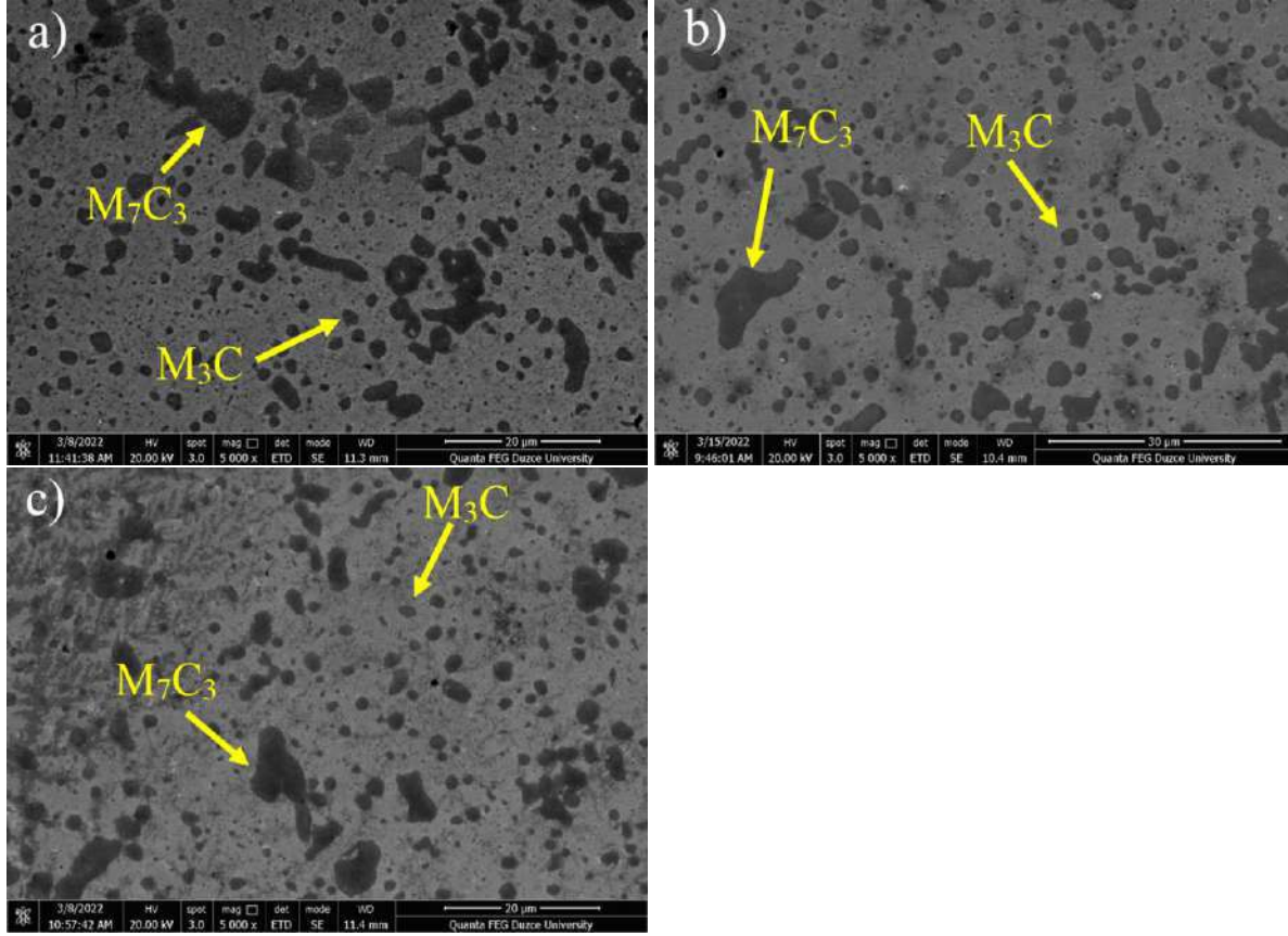
Şekil 4. Farklı ısıl işlem uygulanmış çelik numunelerin SEM görüntüleri a)QT, b) DCT, c) SCT.
