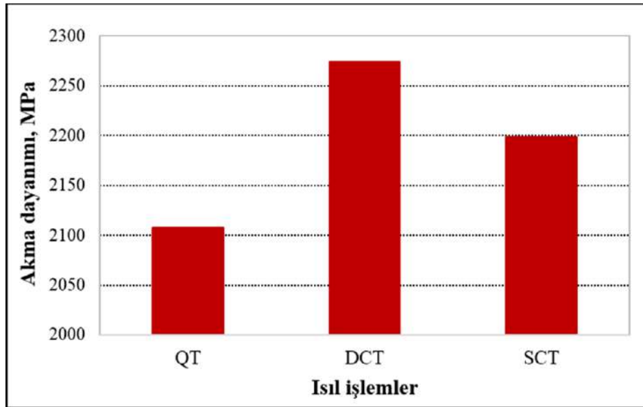
Şekil 7. Farklı ısıt işlem uygulanmış çelik numunelerin akma dayanımı değişim grafiği.
