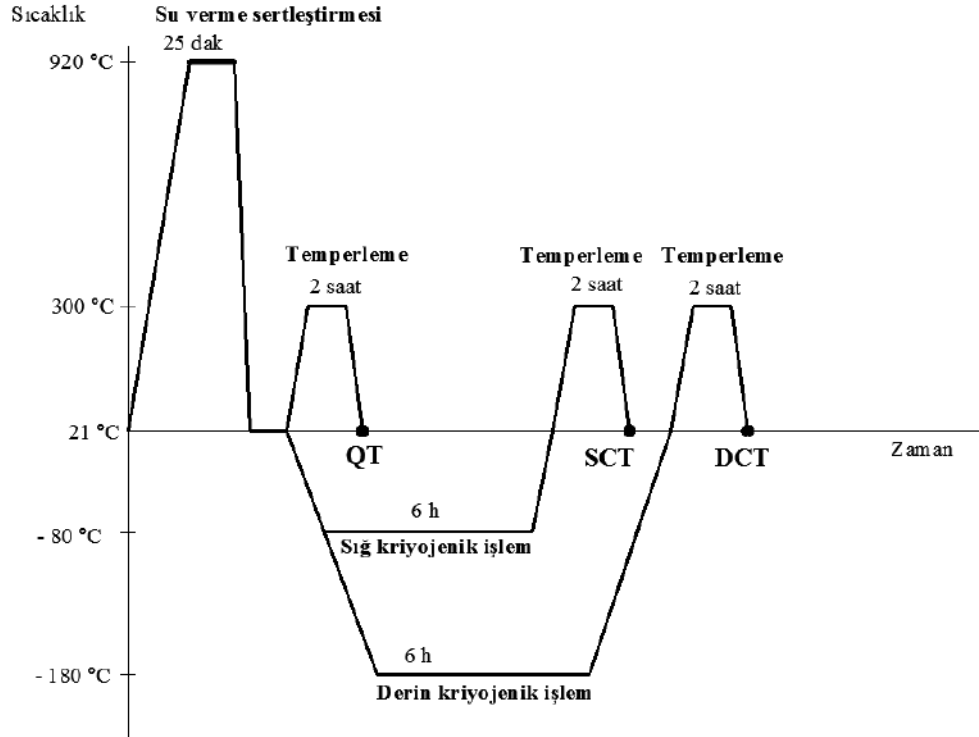
Şekil 1. X210CrW12 soğuk iş takım çeliğine uygulanan ısıt işlemler.
