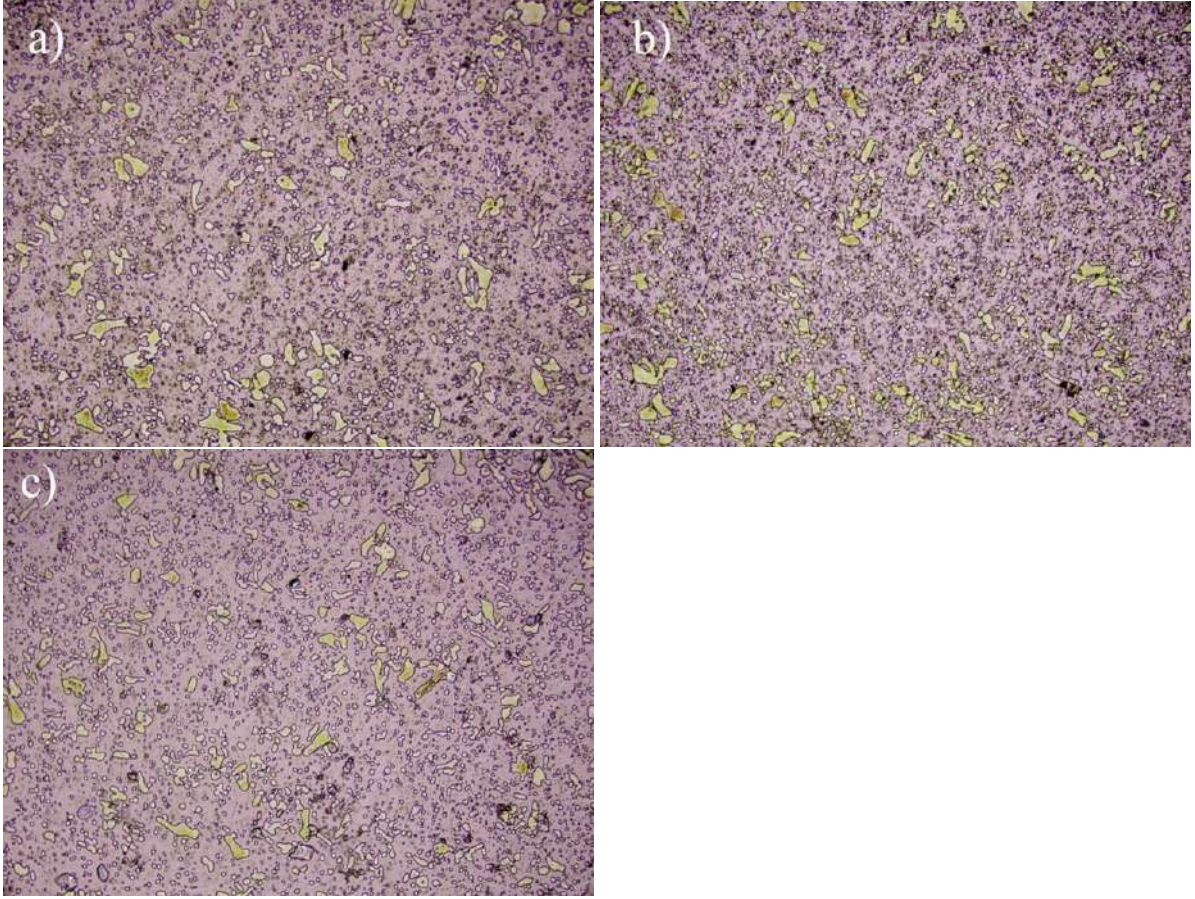
Şekil 3. Farklı ısıtıl işlem uygulanmış çelik numunelerin optik mikroskop görüntüleri a)QT, b) DCT, c) SCT.
